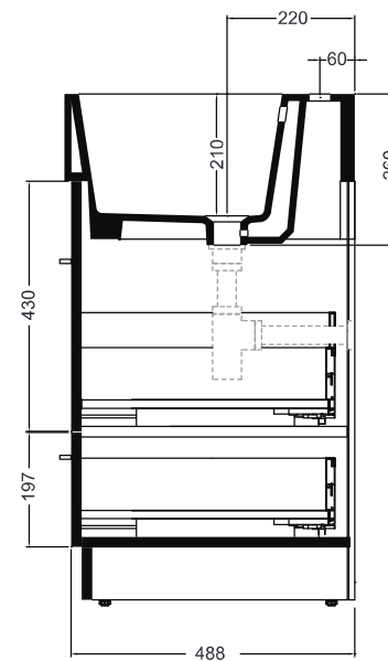
SEZIONE B-B
